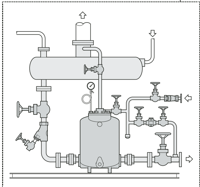
Condensate Recovery Module
